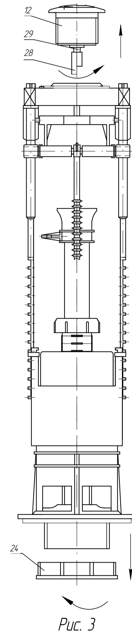
Отвернуть гайку (24) с седла (1) и вывернуть корпус кнопки (12).
