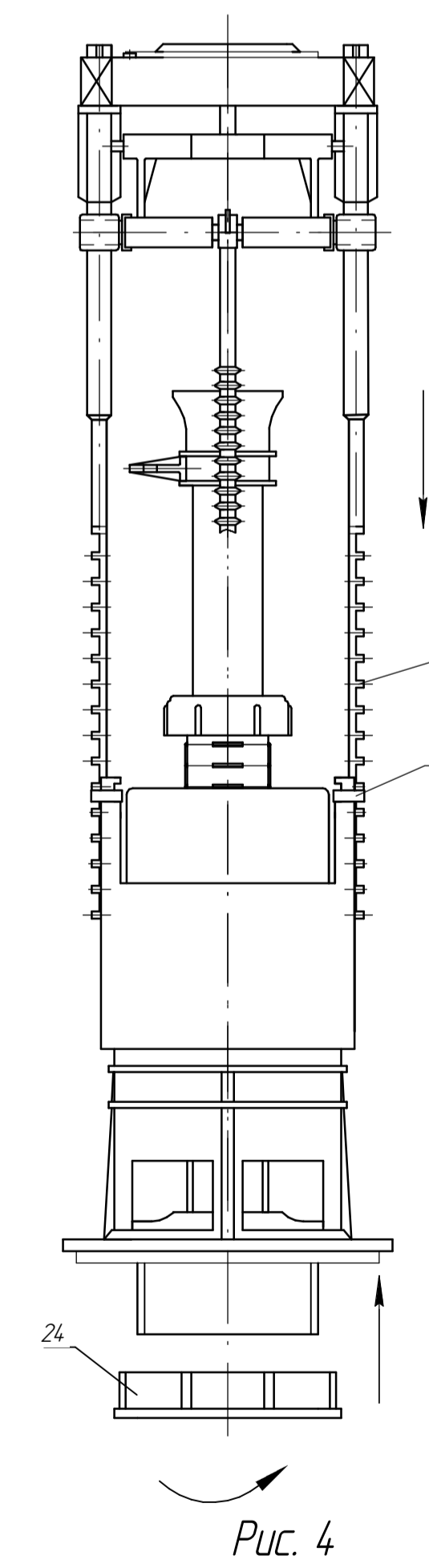
Установить клапан выпуска в бачок и закрепить гайкой (24).
